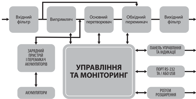
Мал. 7. Блок-схема ДБЖ
