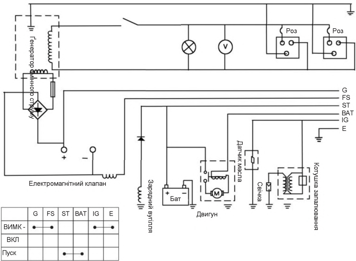
11. ЕЛЕКТРИЧНА СХЕМА
